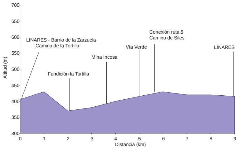
PERFIL SENDERO FUNDICIÓN LA TORTILLA
